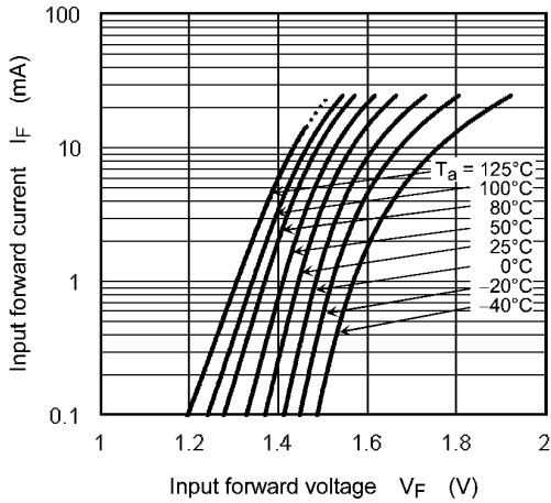
Fig. 12.2.1 I_F - V_F
