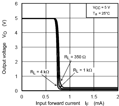
Fig. 12.2.5 V_O - I_F
