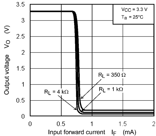
Fig. 12.2.6 V_O - I_F
