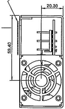
FAN OPTION
